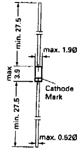
Glass case JEDEC DO-35
